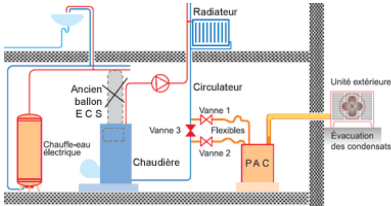
Schéma de raccordement
